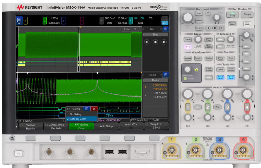
圖 8：在 Keysight InfiniiVision 示波器上執行頻譜分析
